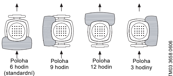
Obr. 5 Polohy svorkovnice
