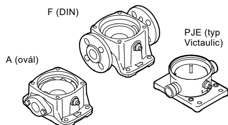
Obr. 13 Přípojky čerpadel
